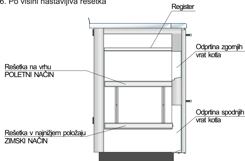
Slika 6. Po višini nastavljiva rešetka
