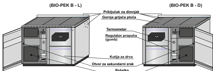
Slika 9. Osnovni dijelovi
