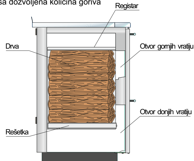
Slika 2. Najviša dozvoljena količina goriva
