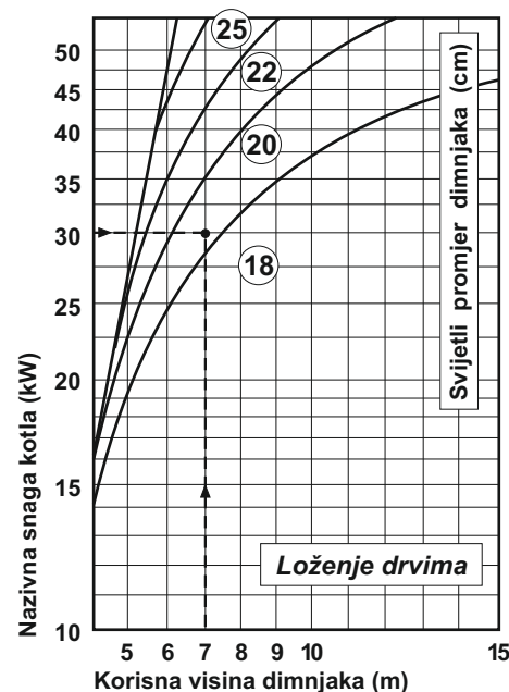
Slika 1. - Dimenzioniranje dimnjaka za kotlove BIO-PEK B
