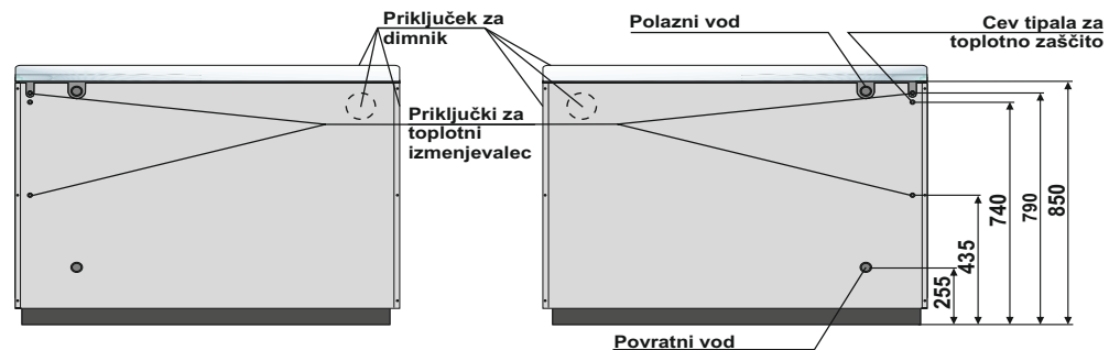
BIO-PEK B - L
