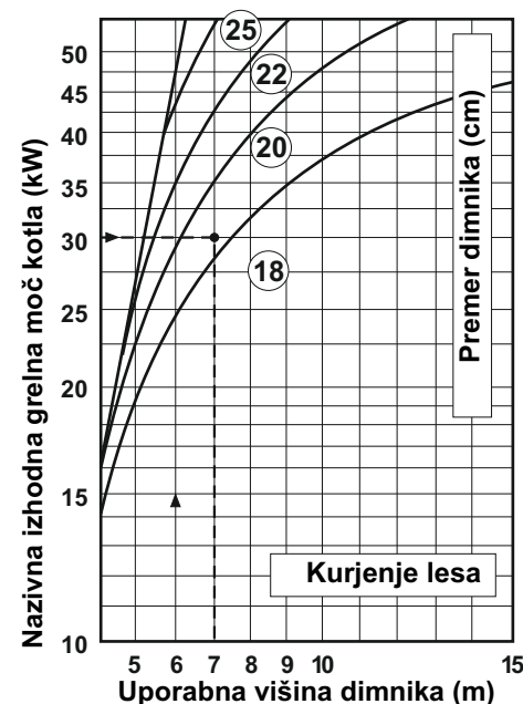
Slika 1. Dimenzije dimnika za BIO-PEK B
