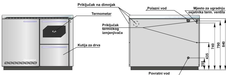
Slika 10. Kotao BIO-PEK B – D (vrijedi i za kotao BIO-PEK B – L)
