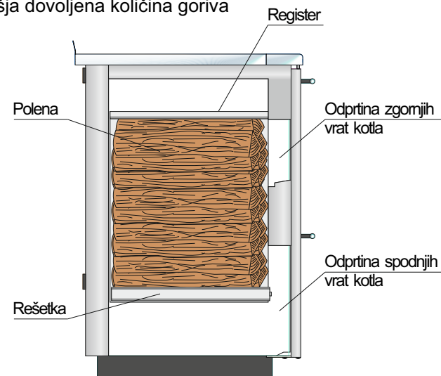
Slika 2. Najvišja dovoljna količina goriva
