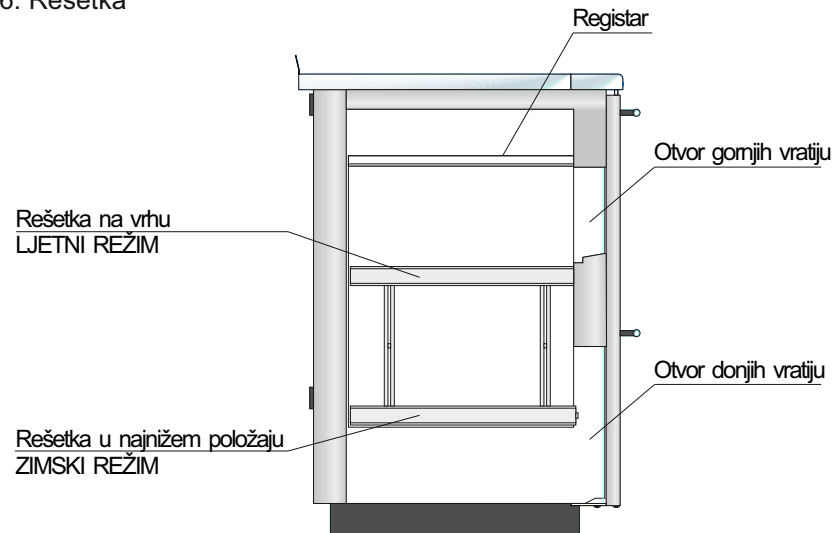
Slika 6. Rešetka
