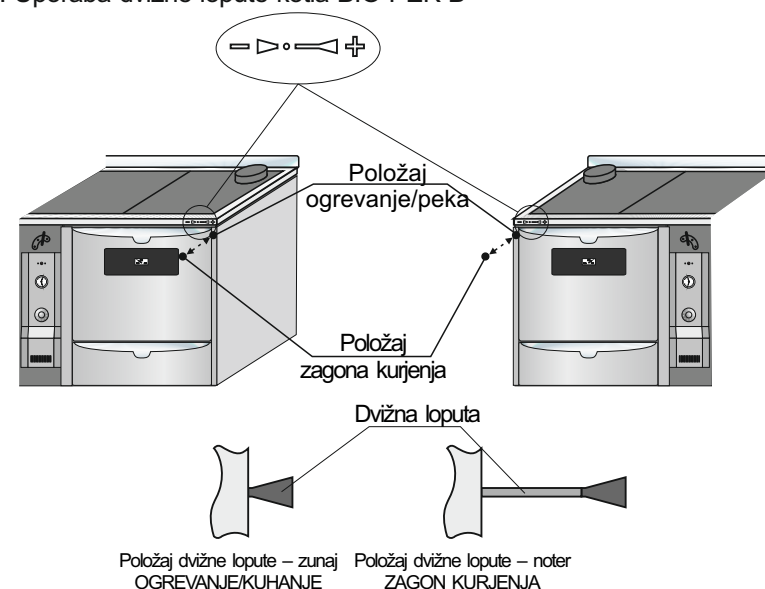
Slika 3. Uporaba dvižne lopute kotla BIO-PEK B
