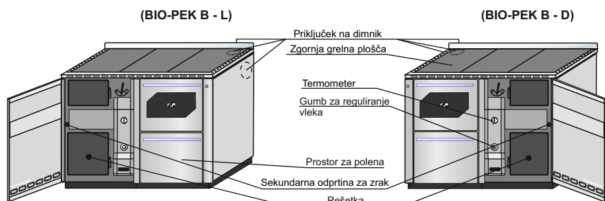
Slika 9. Osnovni deli
