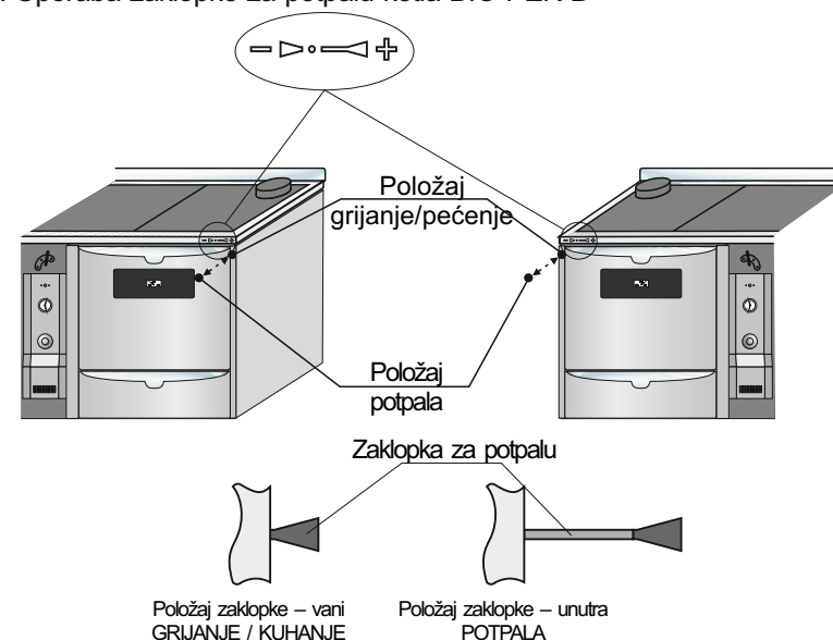
Slika 3. Uporaba zaklopke za potpalu kotla BIO-PEK B
