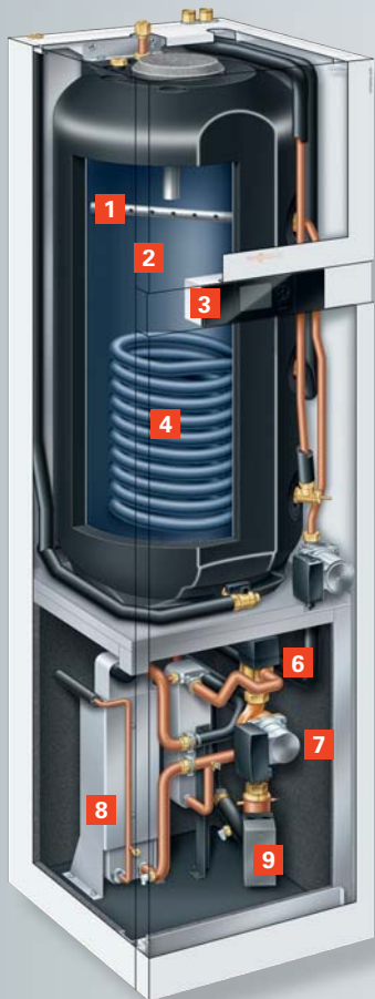
Vitocal 242-S Inneneinheit
