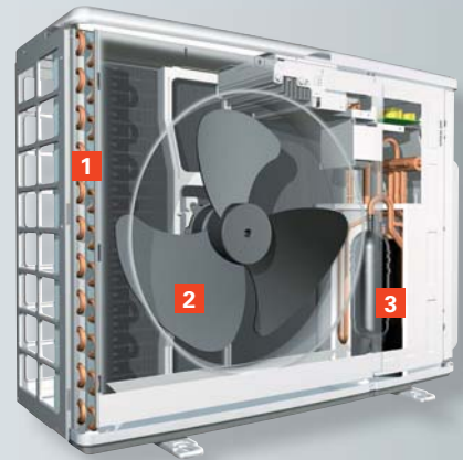
Vitocal 242-S/222-S Außeneinheit
